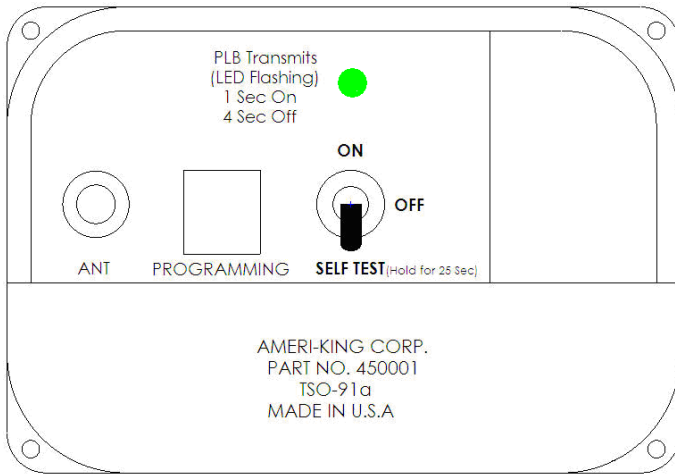
ELT-(S) Top Label
